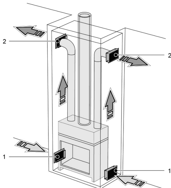
Figuur 21: Ombouw haard met convectiemantel (1) Ventilatievoerrooster, twee openingen van minimaal 175 cm 2 (2) Ventilatie uitstroomrooster, twee openingen van minimaal 175 cm 2
