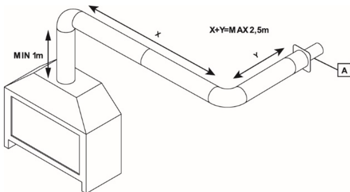
Kanaalconfiguratie 3b
