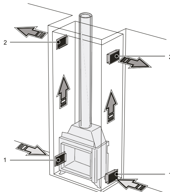
Figuur 20: Ombouw haard zonder convectiemantel (1) Ventilatie toevoerrooster, twee openingen van minimaal 175 cm 2
