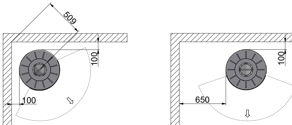
Minimale afstand tot brandbare muur
