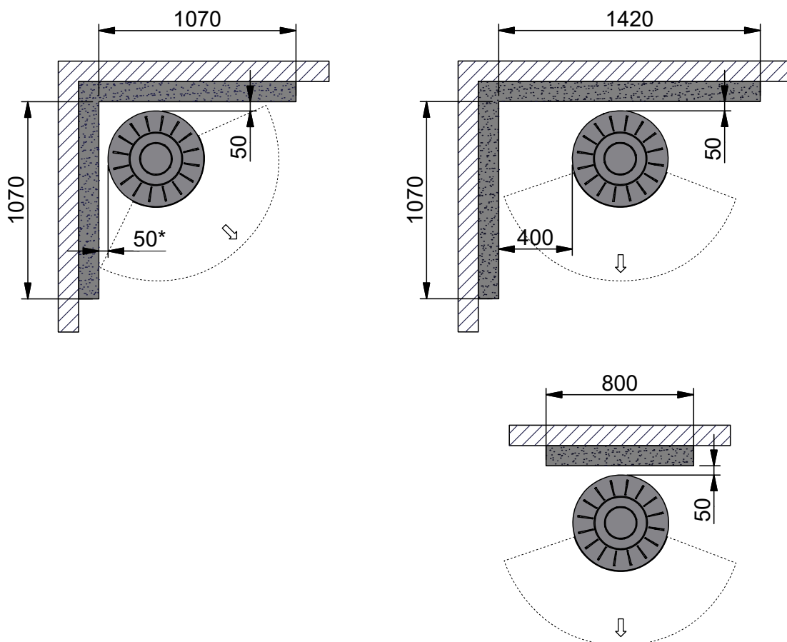
Minimale afstand tot brandbare muur beschermd door brandmuur
