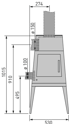
Seitenansicht
