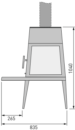
Frontansicht
