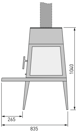
Vooraanzicht
