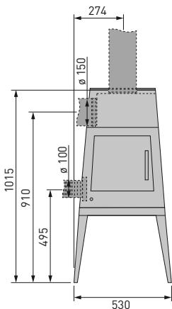
Dimensions en mm
