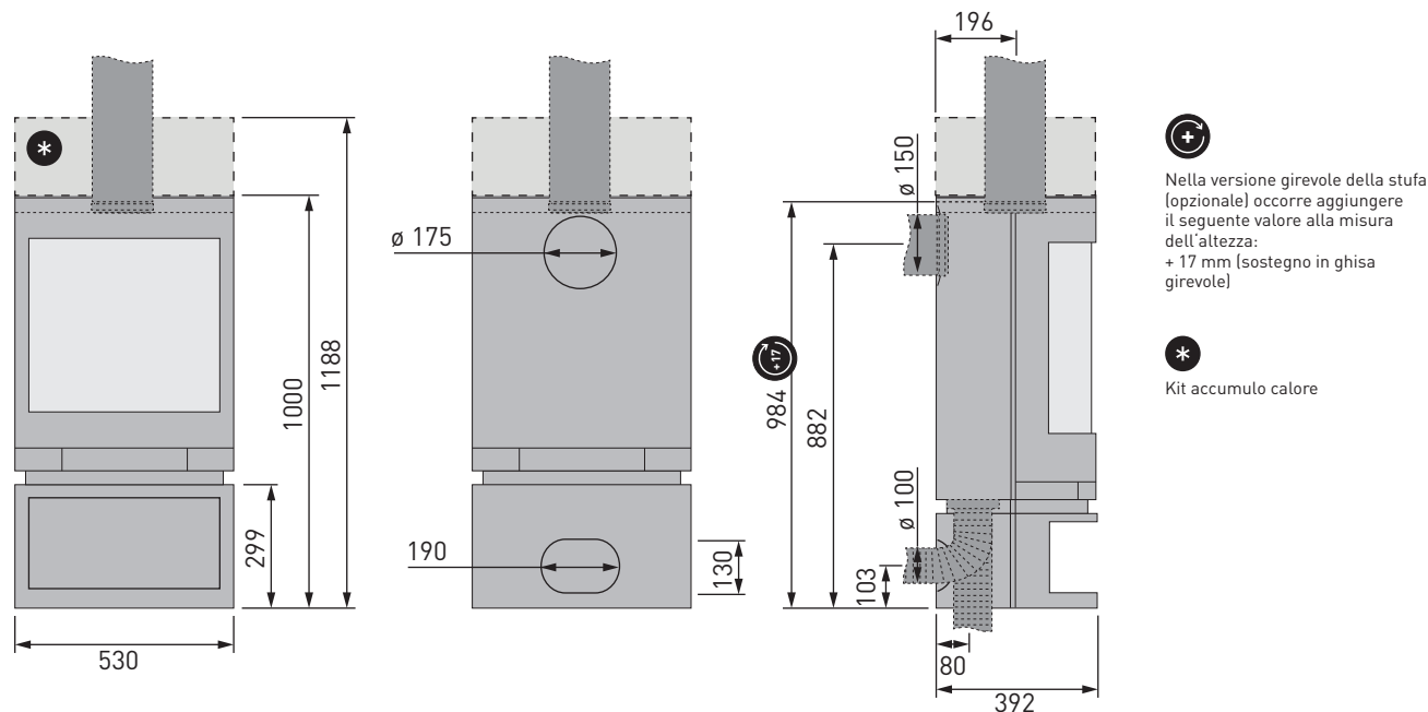
Vista frontale
