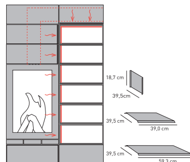
Optik-Tunnel-Box mit eingelegtem Strahlschutzblech
