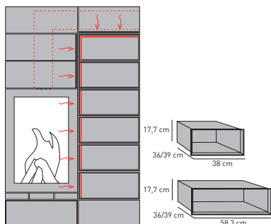
Optik-Box mit Strahlschutzeinsatz
