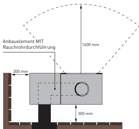
Draufsicht Brennkammer
