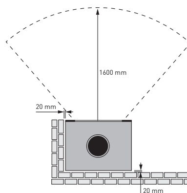
Draufsicht Brennkammer
