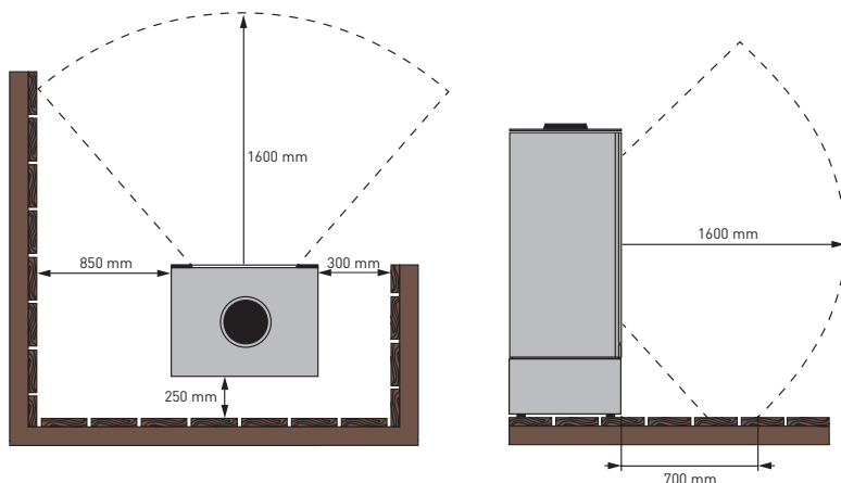
Draufsicht Brennkammer
