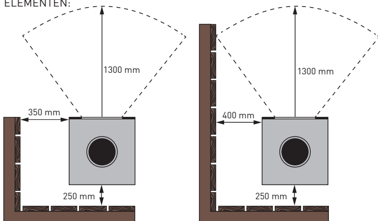
Bovenaanzicht
