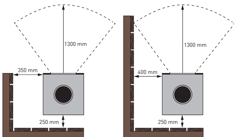
Draufsicht Brennkammer
