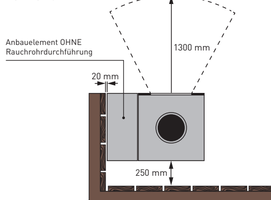
Draufsicht Brennkammer
