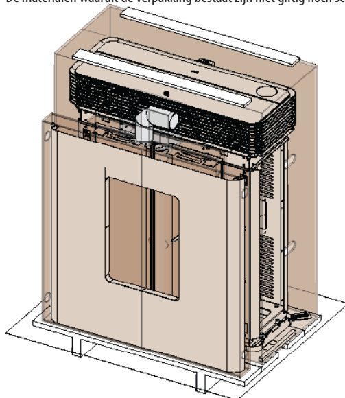
VERPAKKING STRUCTUUR + METALEN BEKLEDING + BOCHT (ACHERUITGANG)
