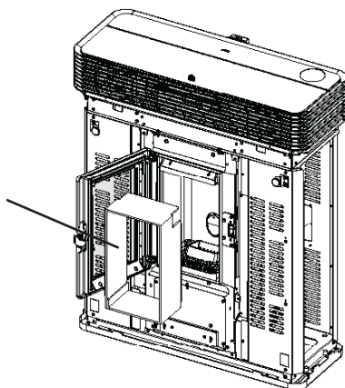
VERPAKKING STRUCTUUR + METALEN BEKLEDING + BUIS (BOVENUITGANG UP!)
