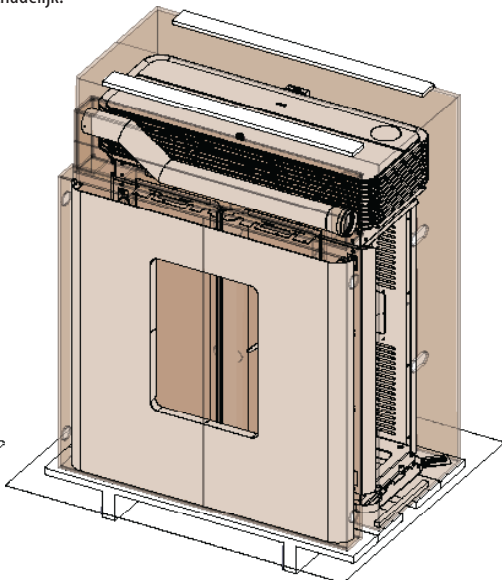
VERPAKKING STRUCTUUR + METALEN BEKLEDING + BUIS (BOVENUITGANG UP!)
