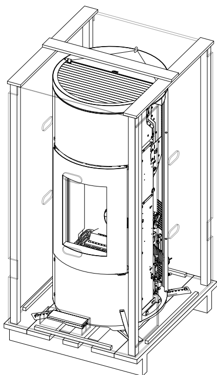
VERPAKKING STRUCTUUR KACHEL
