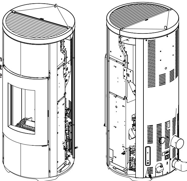
KACHEL ZONDER BEKLEDING
