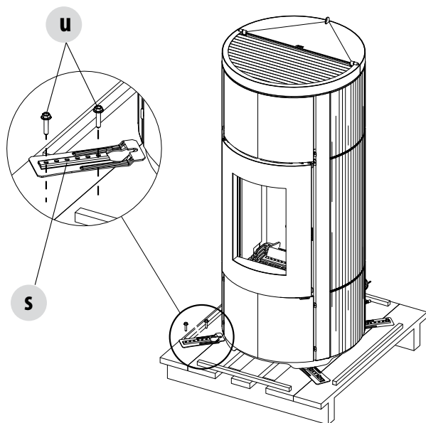
VERWIJDERING BEVESTIGINGSBEUGELS
